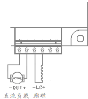
他励直流电机输出接线图
