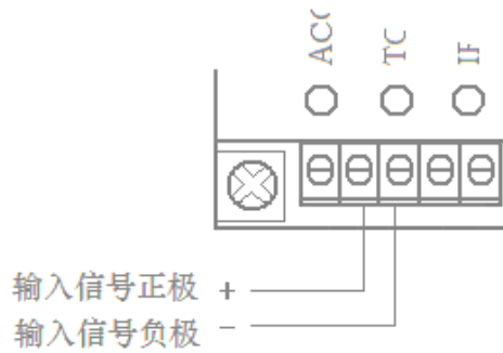
AL型产品外部信号输入说明
