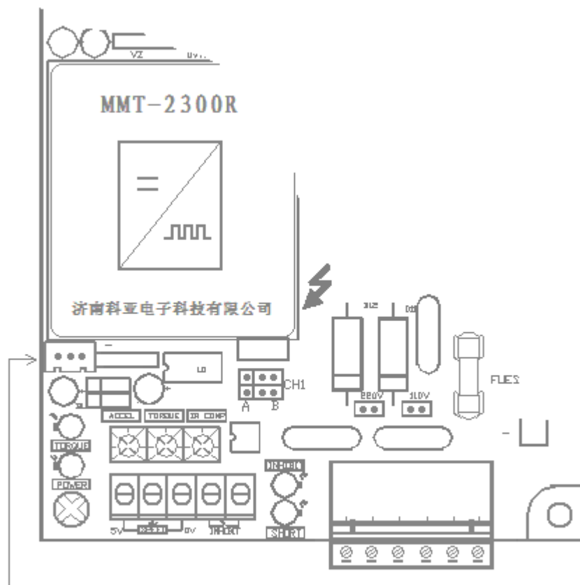
专用外置VID接口 BL型产品信号经隔离器送VID接口说明
